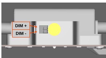
Anschlussbelegung des Dimmeingangs
